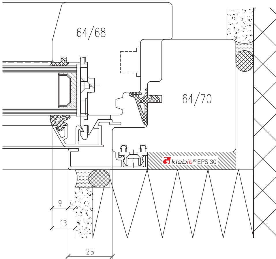
Fenster-Flügel, Anschluss seitlich
